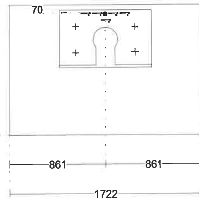
Ansicht C
