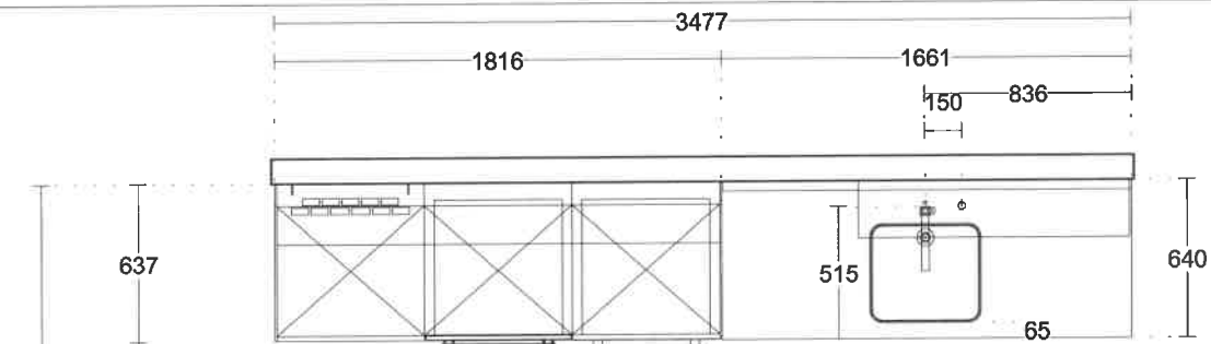
Ansicht A
